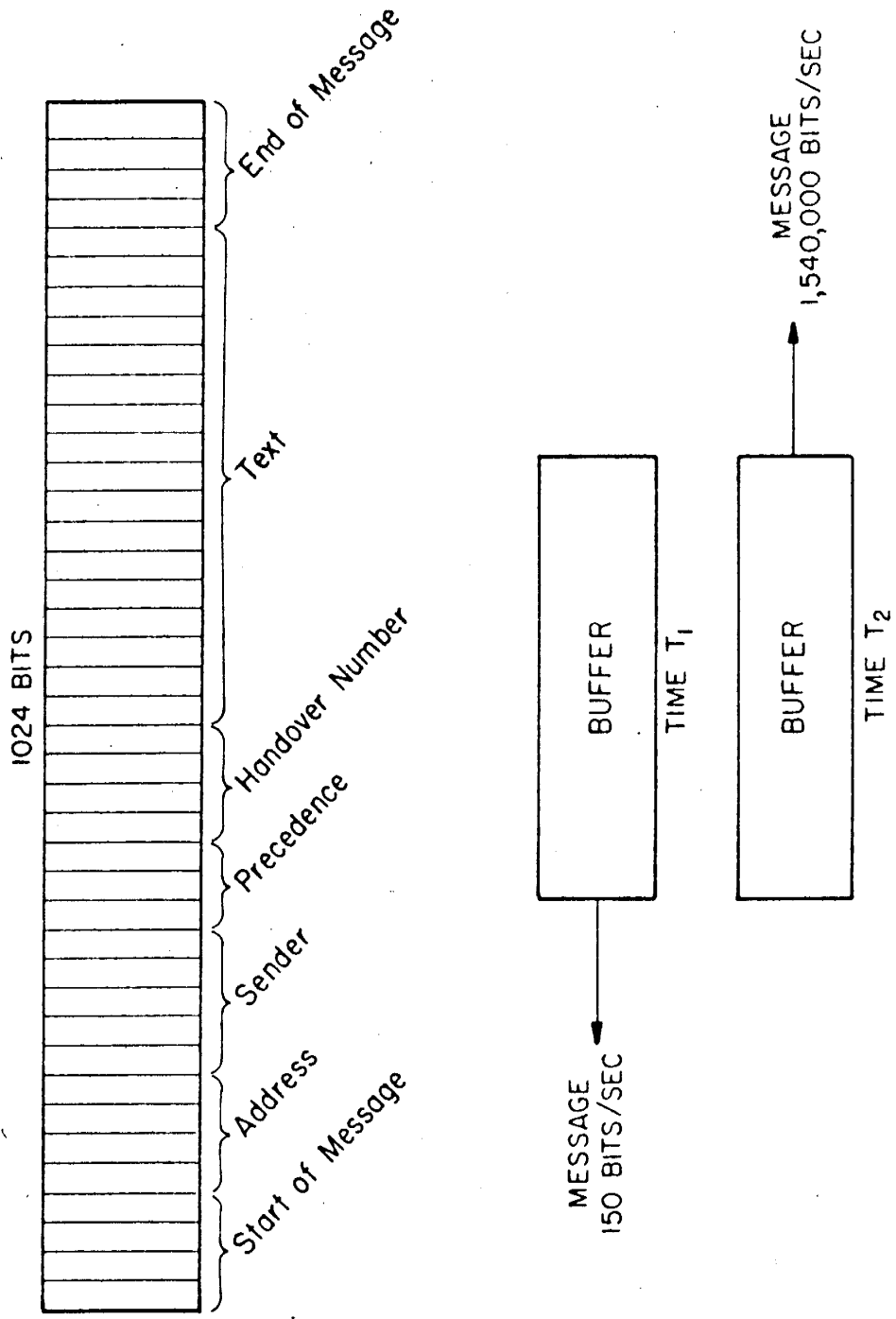
FIG. 10 — Message Block
